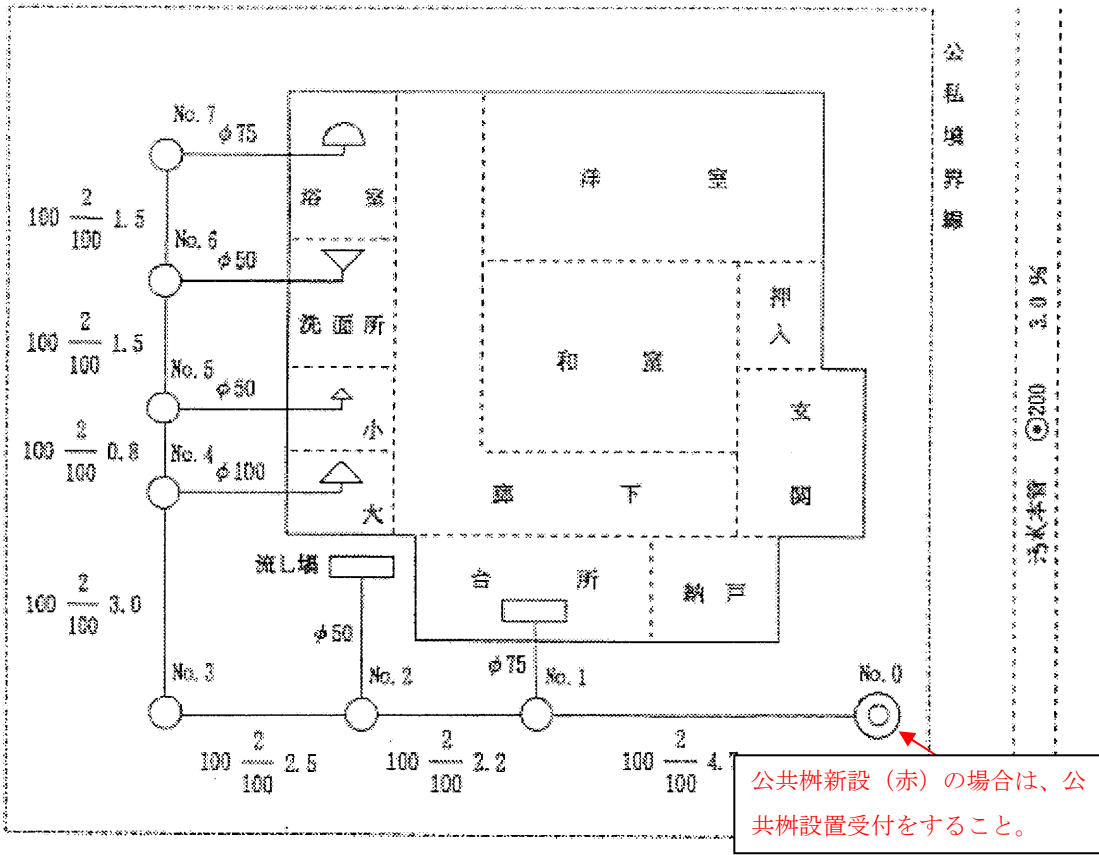
平面図 S=1/100
