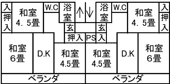
< 住宅平面図 >
