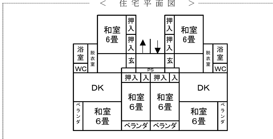
< 住宅平面図 >
