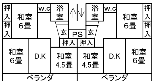
< 住宅平面図 >
