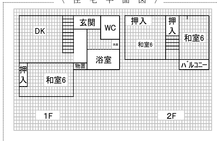
〈 住 宅 平 面 図 〉
