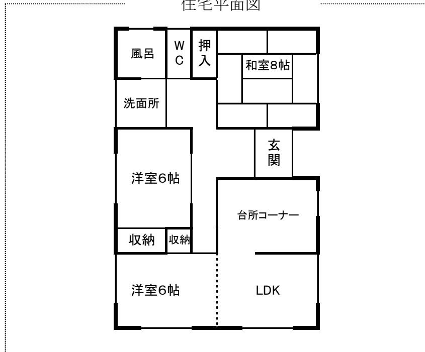
住宅平面図
