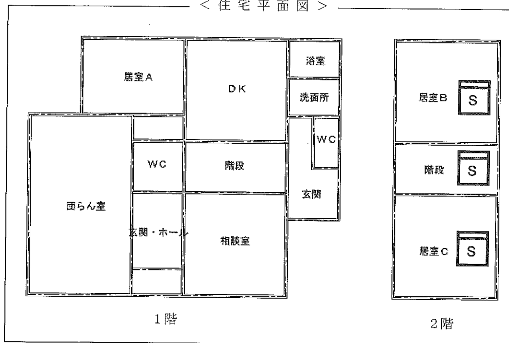
< 住宅平面図 >
