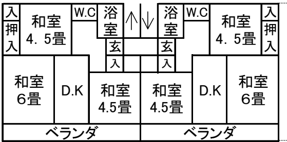
< 住宅平面図 >
