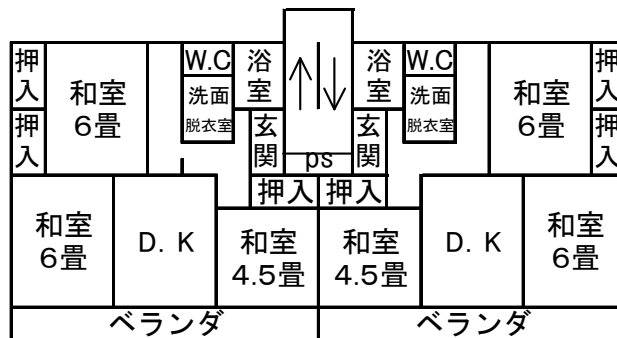
< 住 宅 平 面 図 >
