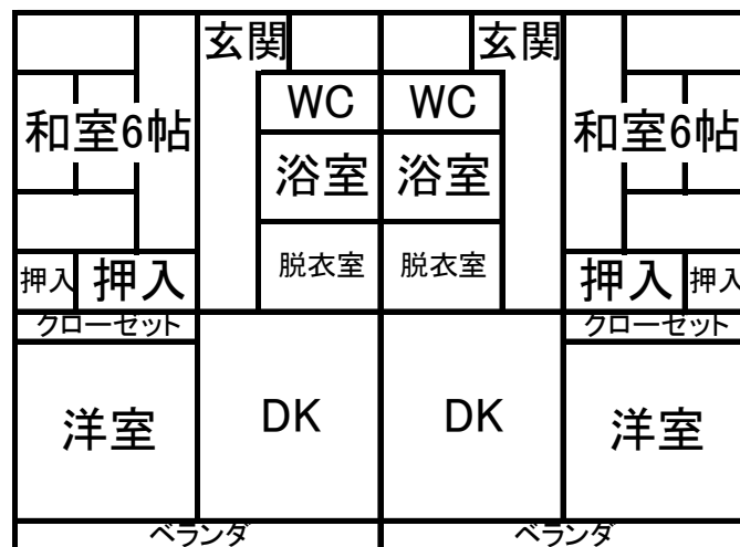
< 住宅平面図 >
