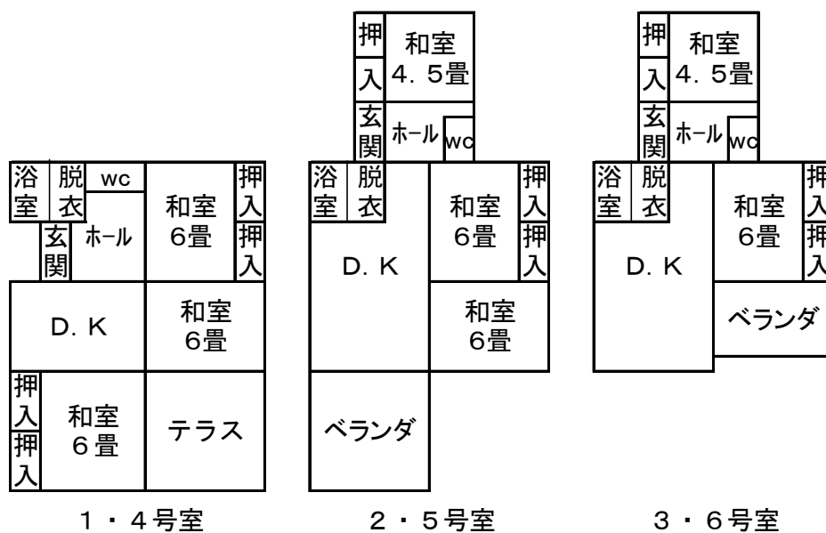
< 住宅平面図 >
