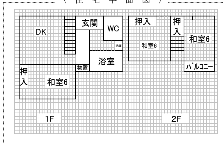
〈 住 宅 平 面 図 〉
