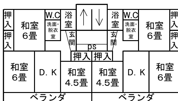
< 住宅平面図 >
