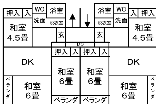
< 住 宅 平 面 図 >
