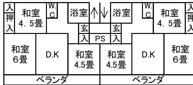
< 住宅平面図 >
