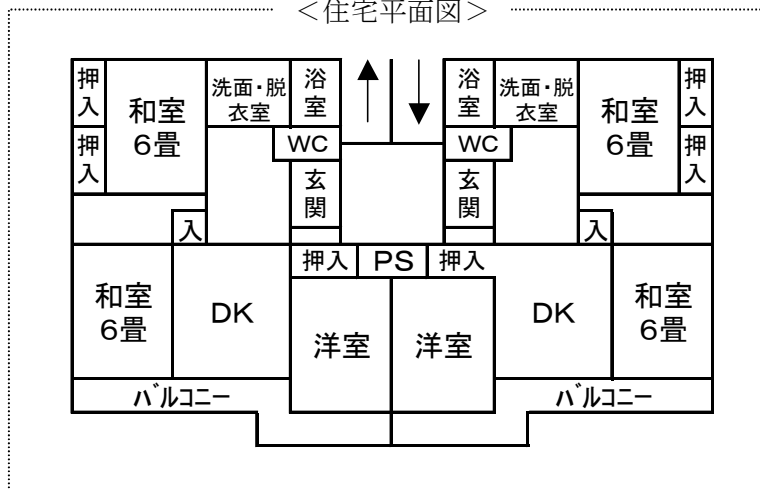
<住宅平面図>
