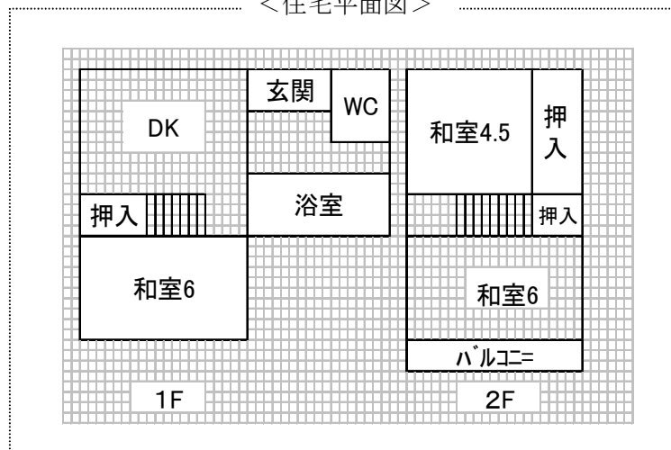
<住宅平面図>
