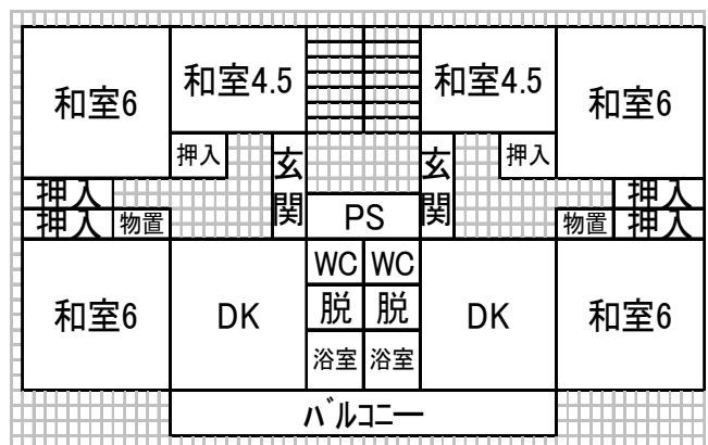
<住宅平面図>
