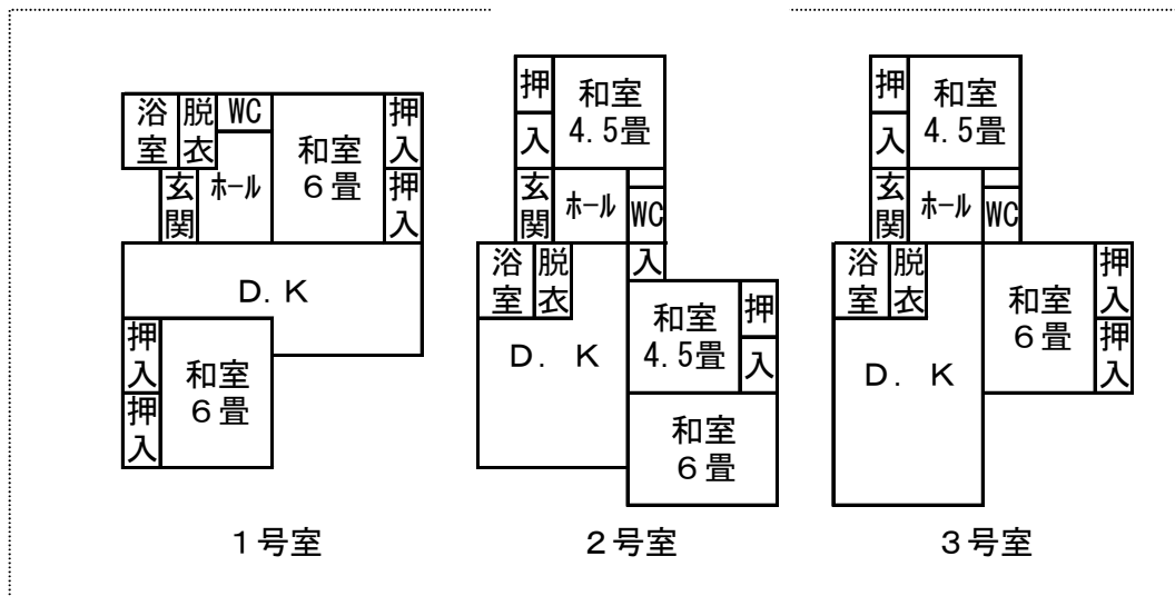
<住宅平面図>
