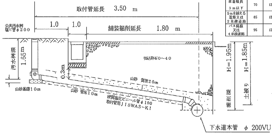
断面図
