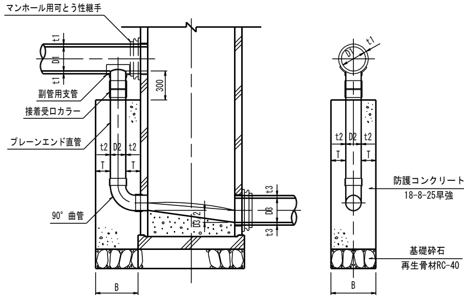
副管詳細図
