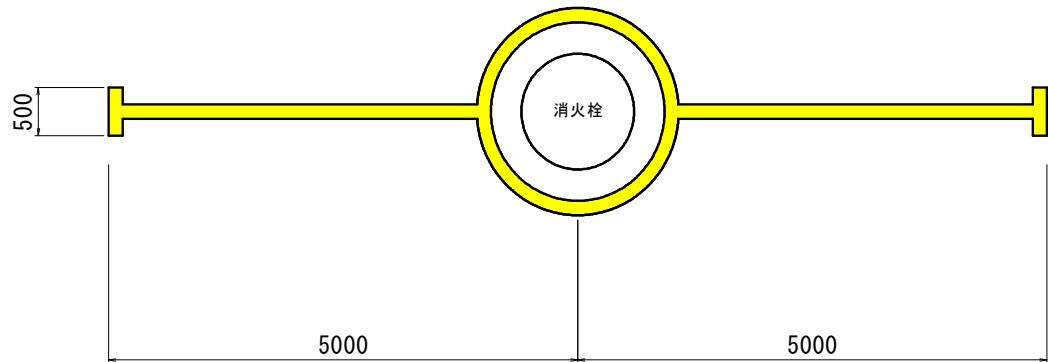
消火栓(円形)
