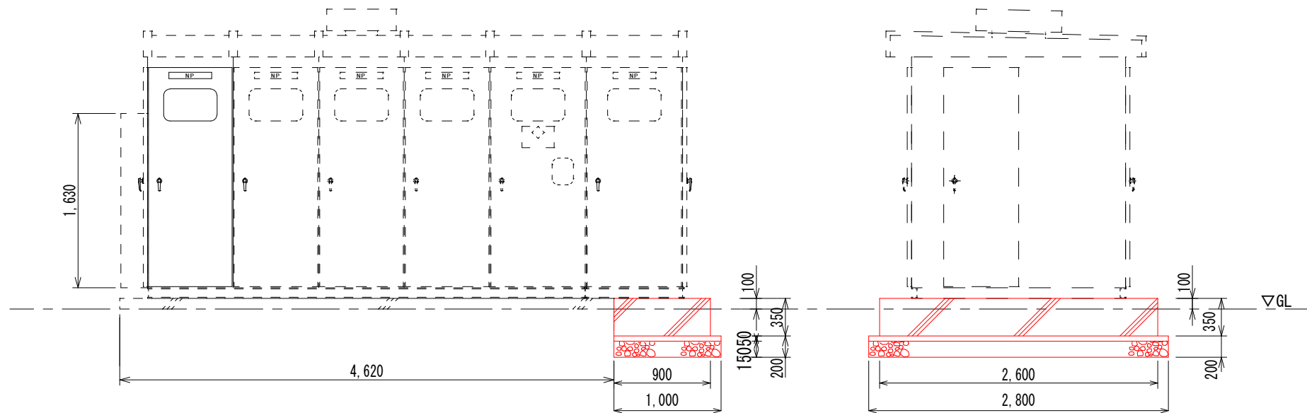
基礎図（改修後） (S=1/50)
