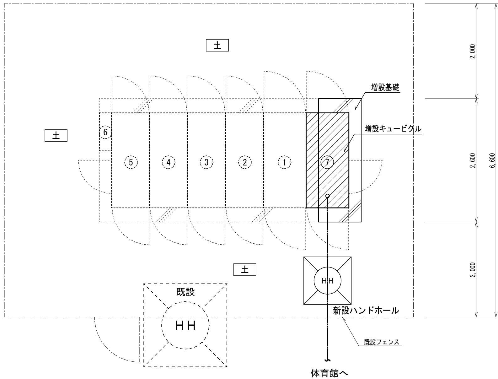
屋外キュービクル平面図（改修後）（S=1/50）
