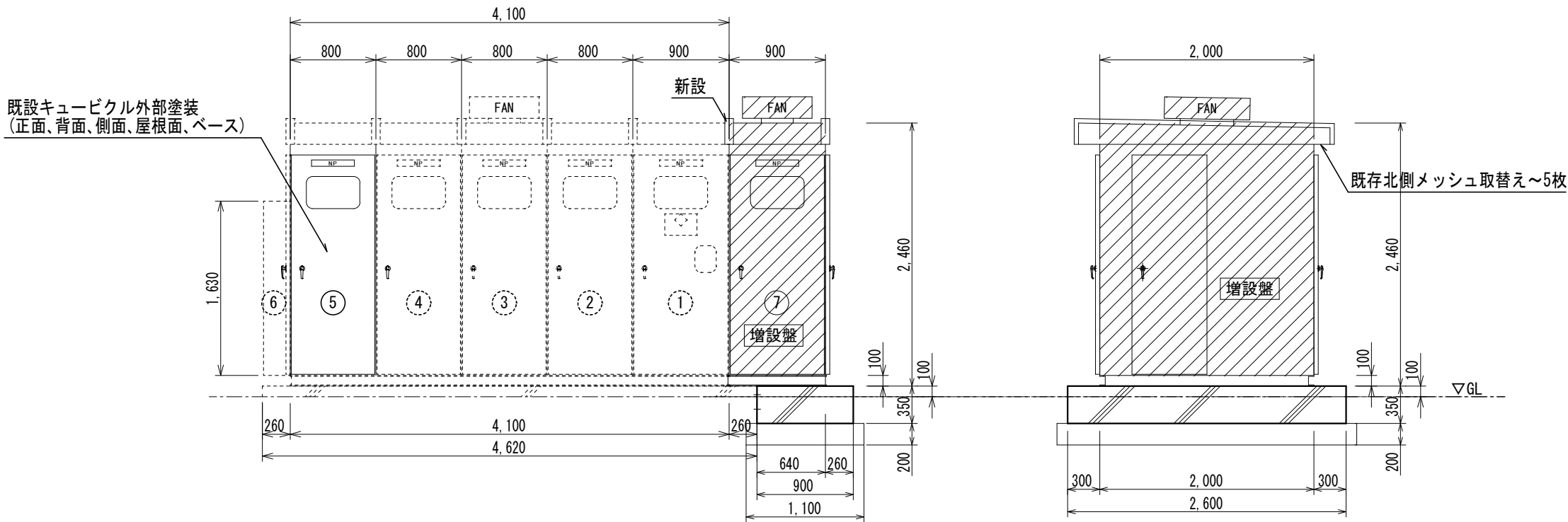
屋外キュービクル参考姿図（改修後）（S=1/50）
