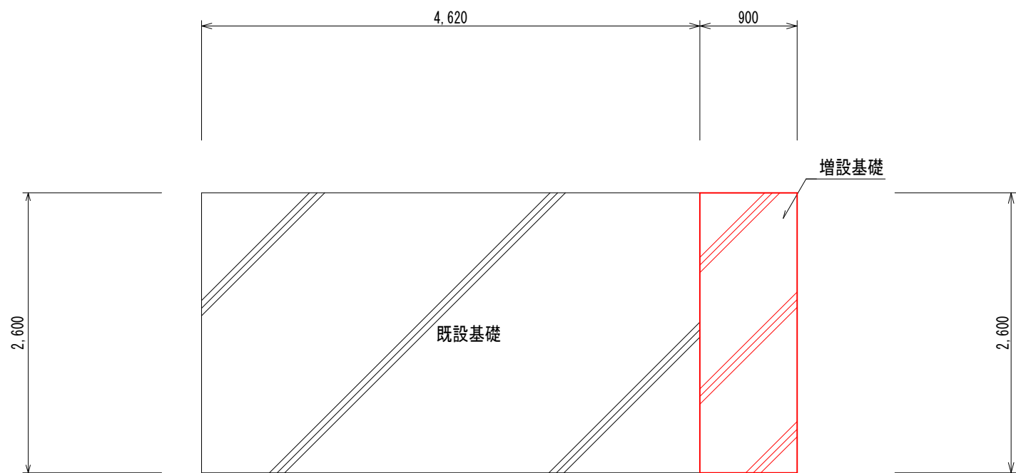
基礎平面図（改修後） (S=1/50)
