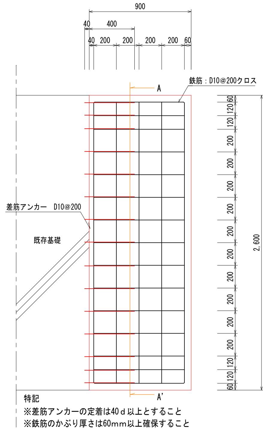
基礎構造図 (S=1/20)
