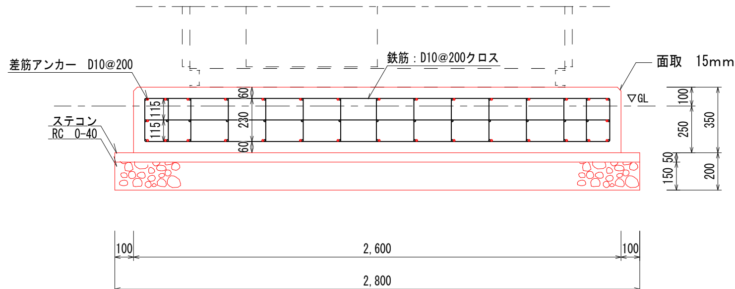
A-A' 断面図 (S=1/20)
