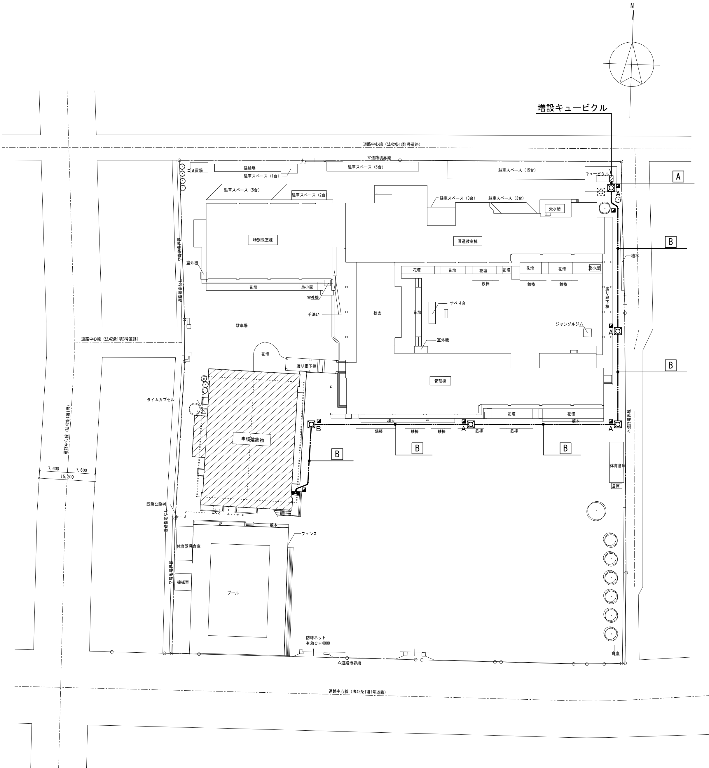
配置図 S=1:600
