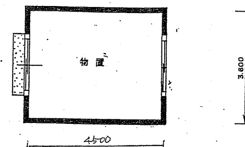
物置平面図
